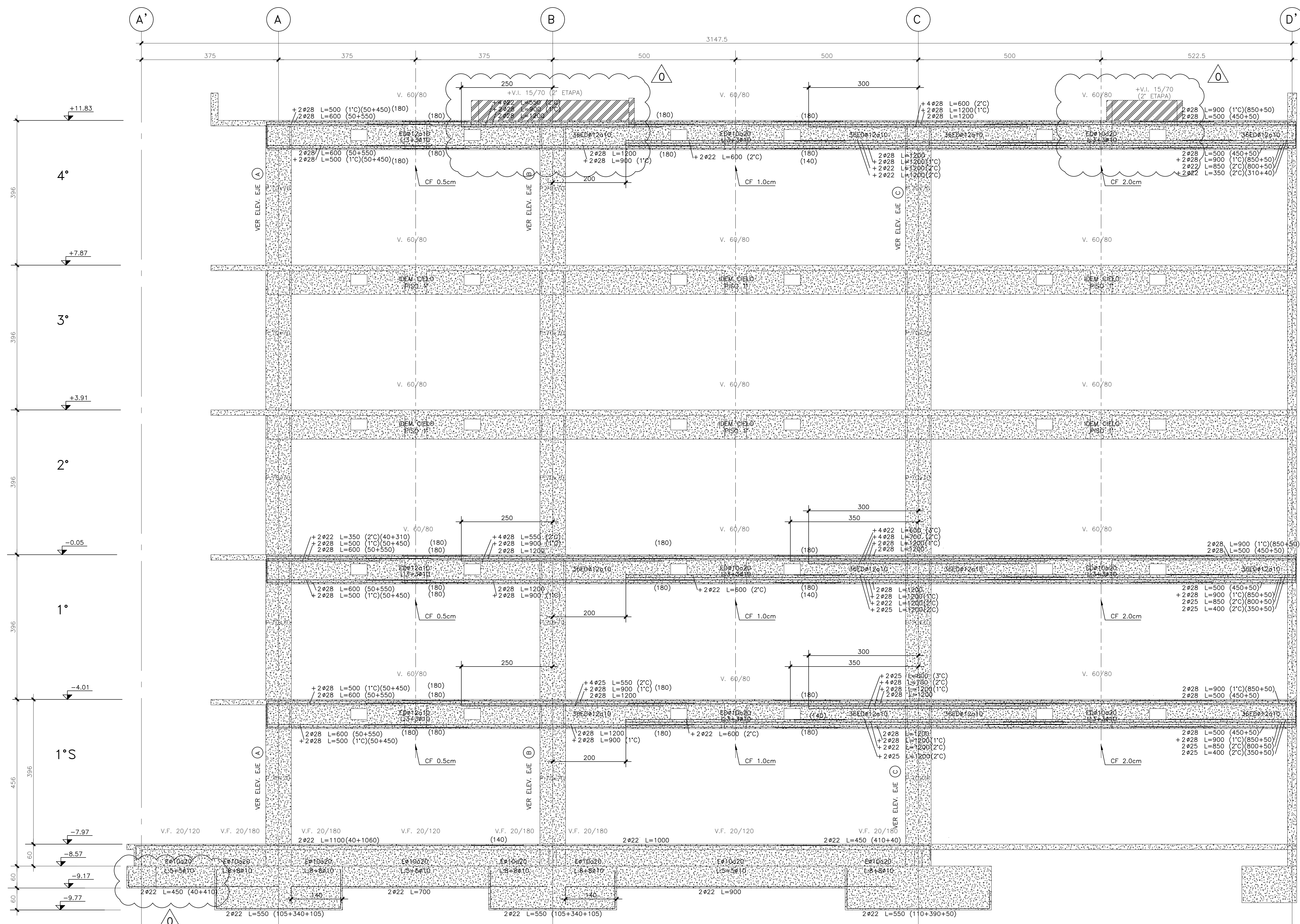
ELEVACION EJE 2 ESCALA 1:50
